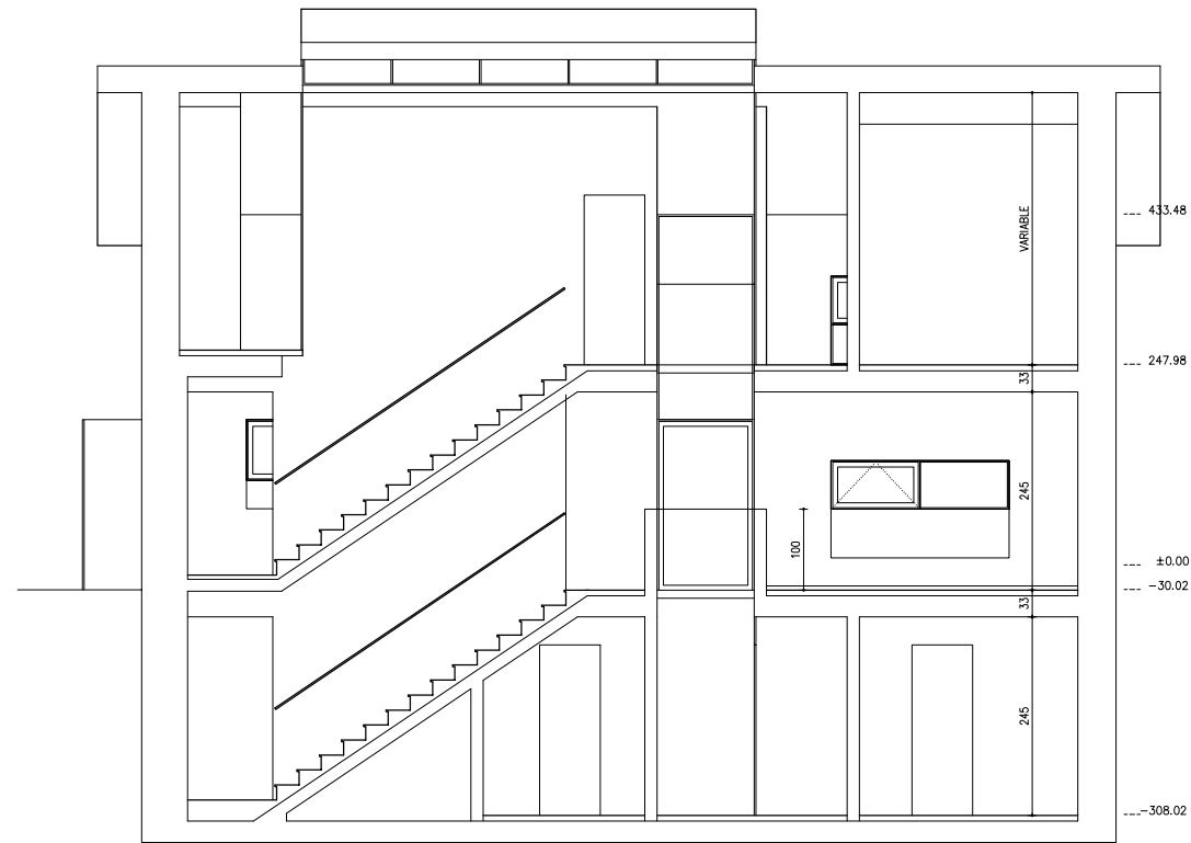
SECCION 4-4
