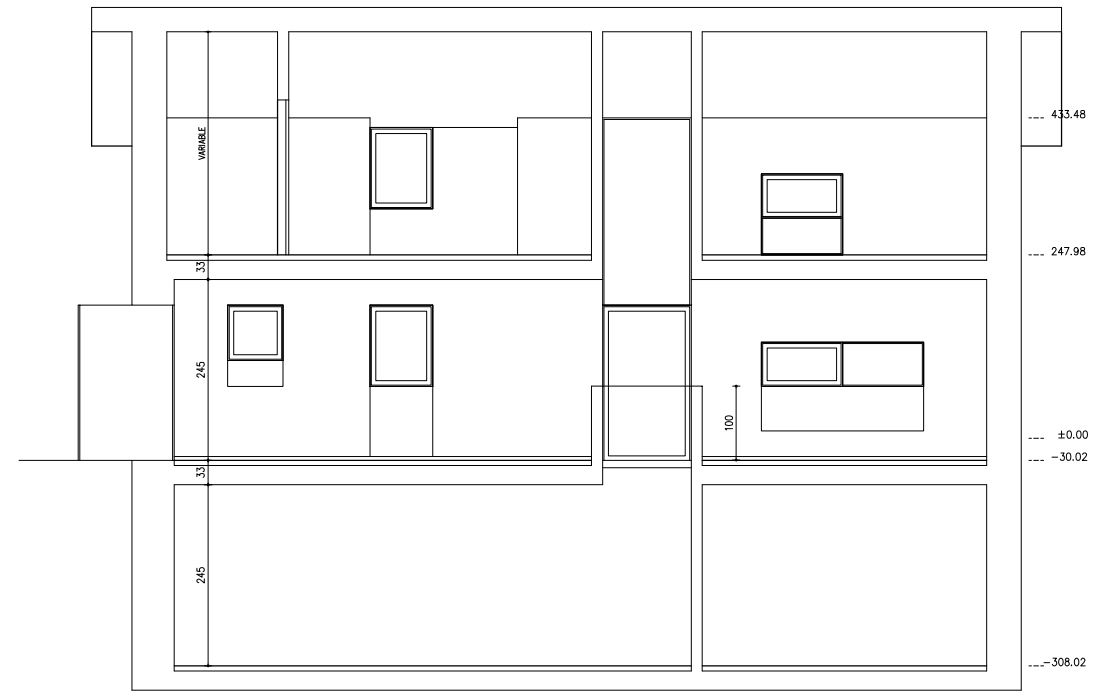
SECCION 5-5
