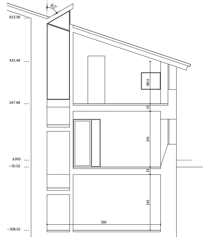
SECCION 7-7
