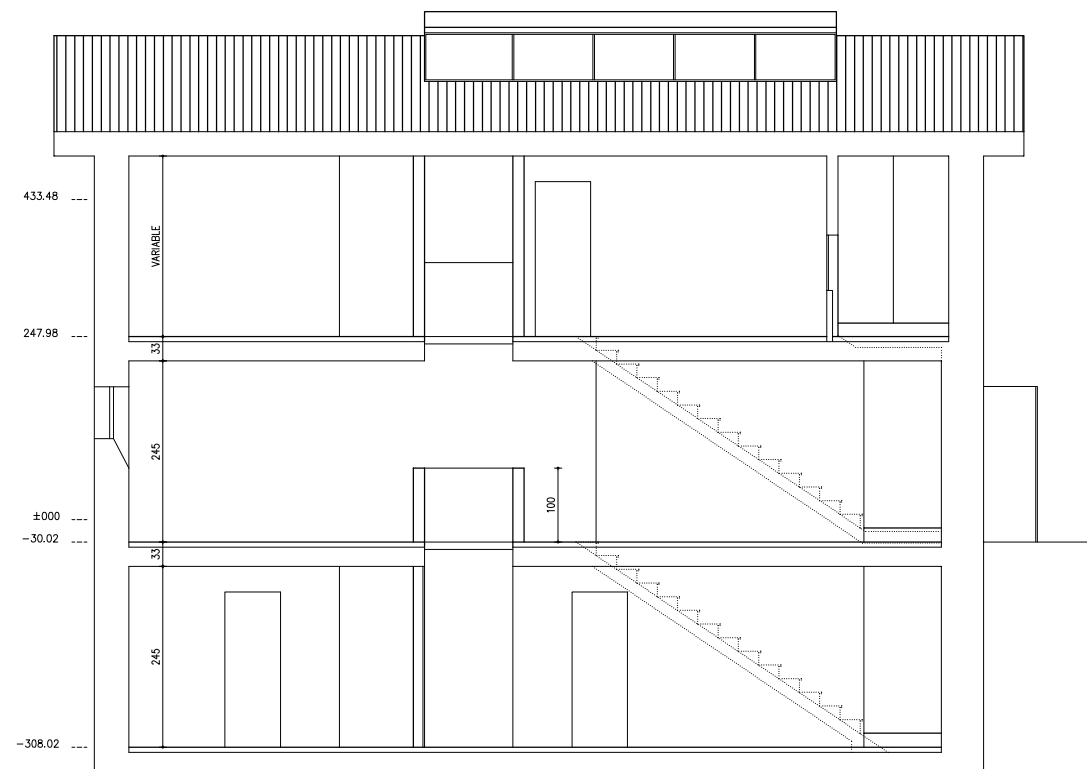
SECCION 6-6
